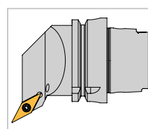
HSK-T63- SV117,5CL/R 45070-16
