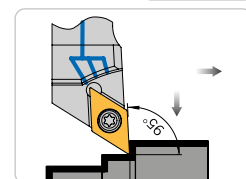
Right holder and right module shown Adattatore destro e modulo destro in figura Support droit et module droit montés
